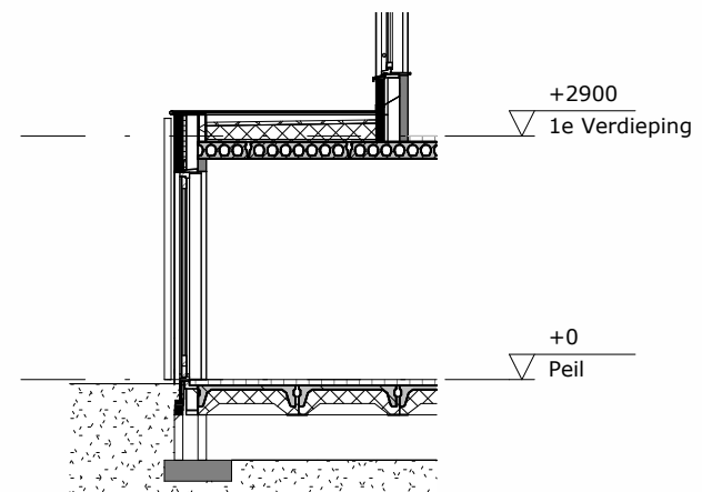
Doorsnede schaal 1 : 100
