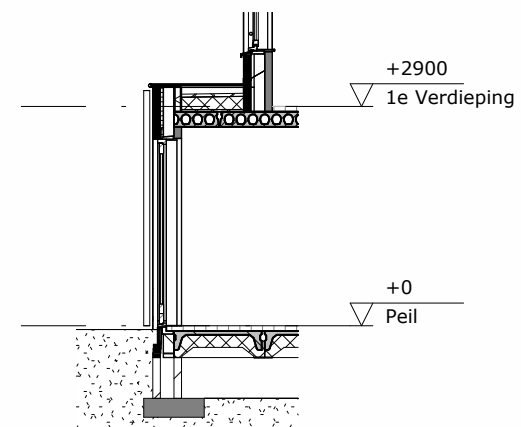
Doorsnede schaal 1 : 100
