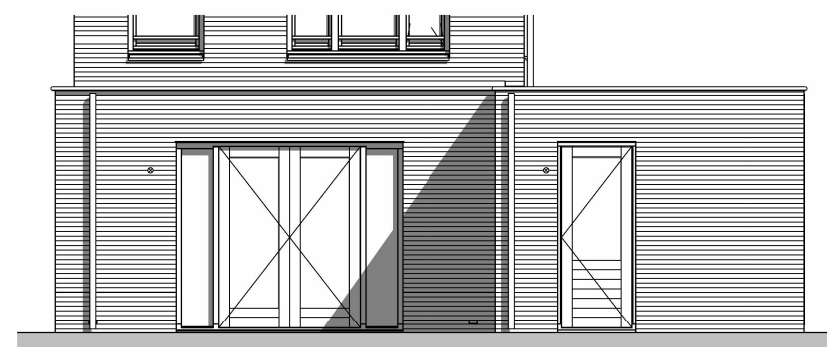
Achtergevel schaal 1 : 100
