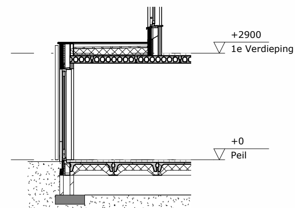
Doorsnede schaal 1 : 100
